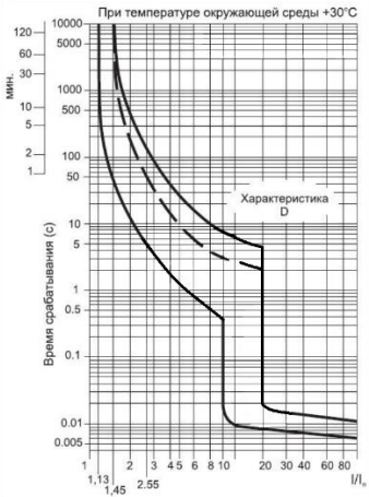
Рис. 2 Время-токовая характеристика С
