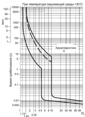
Рис. 1 Время-токовая характеристика С
