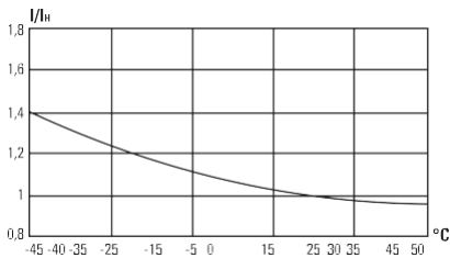
Рис. 3 Температурный коэффициент
